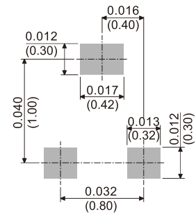
SOT-723
