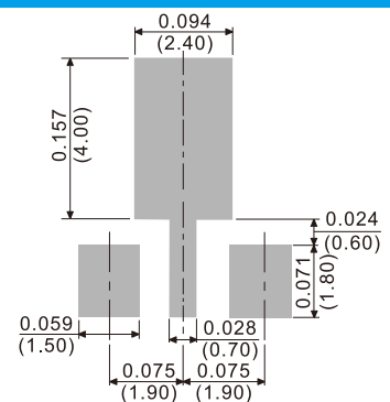
SOT-89
