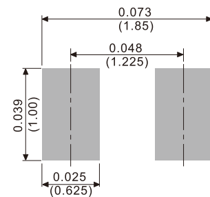
DFN1610-2L
