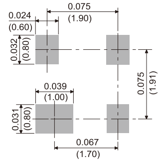
SOT-143
