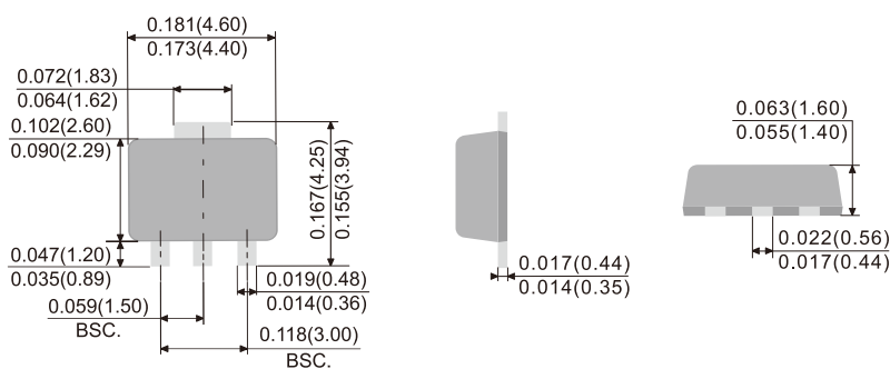
SOT-89
