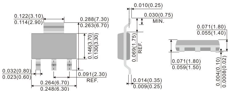
SOT-223
