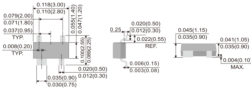
SOT-143
