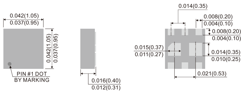
DFN1010B-6L
