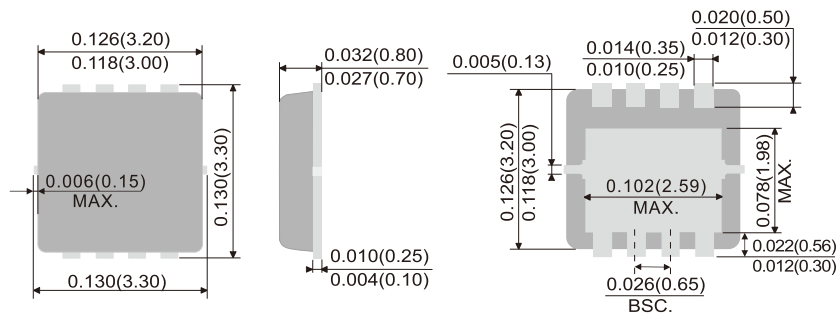
DFN3333-8L
