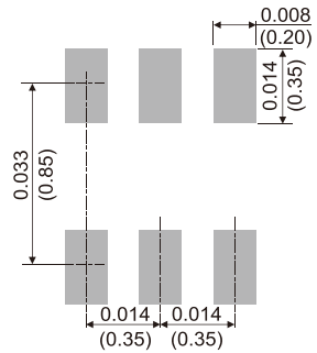
DFN1010B-6L
