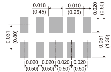
DFN3810-9L
