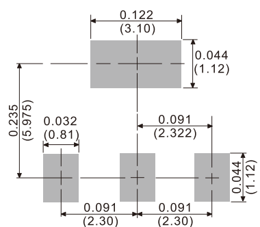
SOT-223
