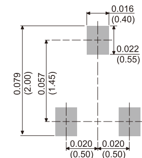
SOT-523
