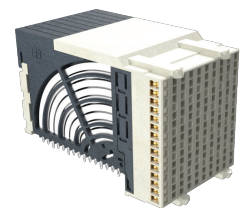
Right Angle Receptacle
